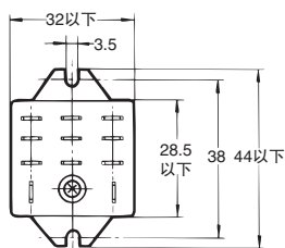
安装孔加工尺寸
