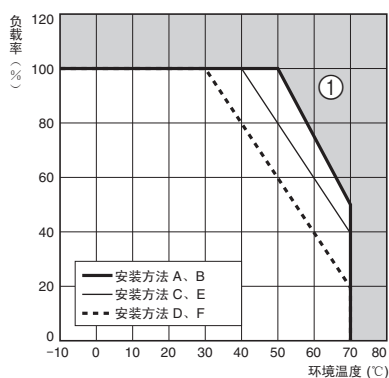
附带底板型 (150W)
