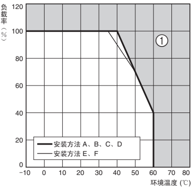
附带底板・罩盖型（30W）
