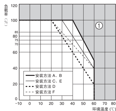
附带底板·罩盖型 (150W)
