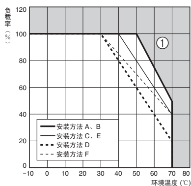
附带底板·罩盖型 (240W)
