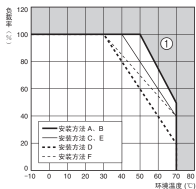
开放、附带底板型 (240W)
