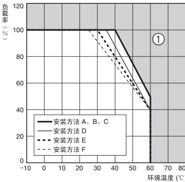
附带底板・罩盖型（50W）
