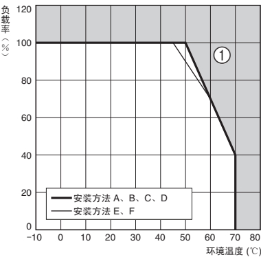
开放型、附带底板型（30W）
